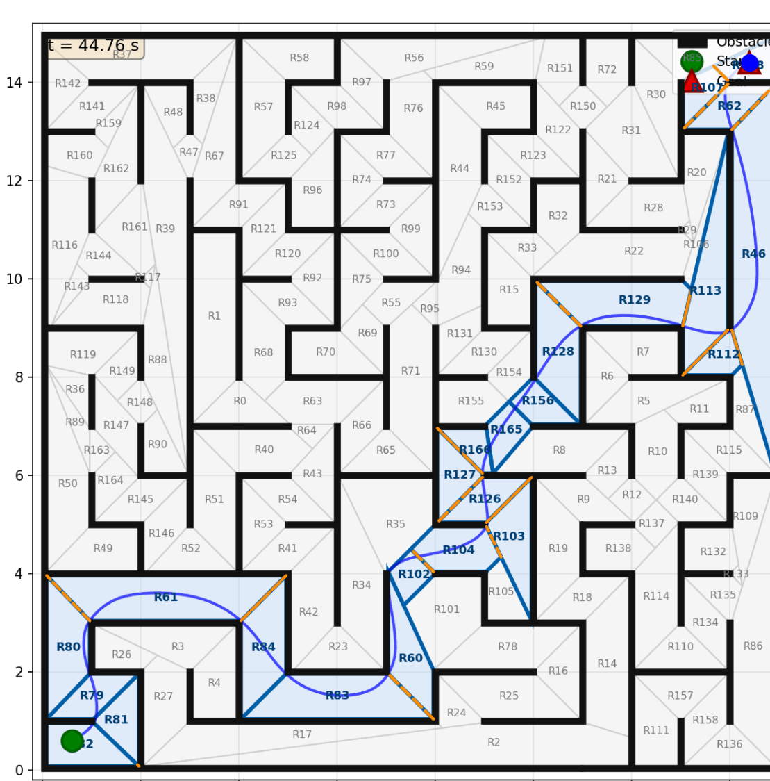
(a) Quỹ đạo GCS-DMS trên mê cung 15 \times 15 . (b) Hồ sơ vận tốc |v| theo thời gian.
